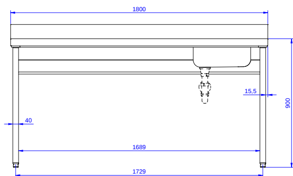
Boční
